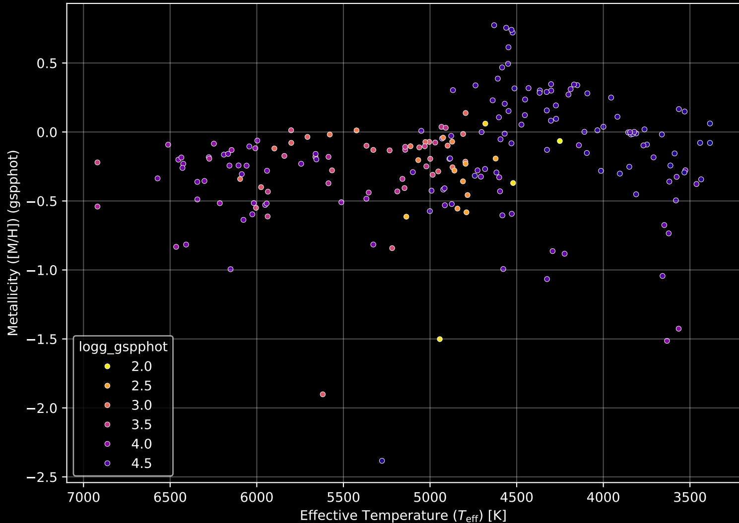
APOGEE DR17 Field: [210+75] Stellar Population Parameters (n= 204)
